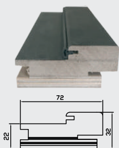
Стойка короба компланарная
