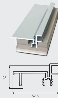
Стойка короба скрытая алюминиевая
