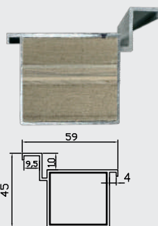
Стойка короба скрытая алюминиевая универсальная
