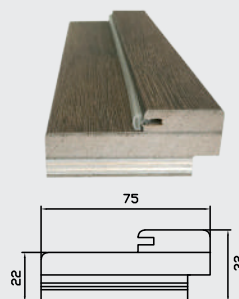
Стойка короба комбинированная
