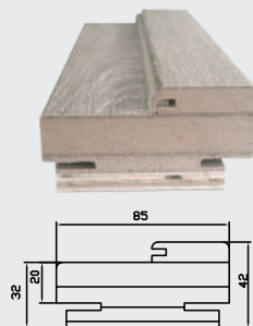
Стойка короба серии Альфа
