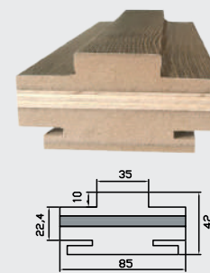
Стойка короба барная
